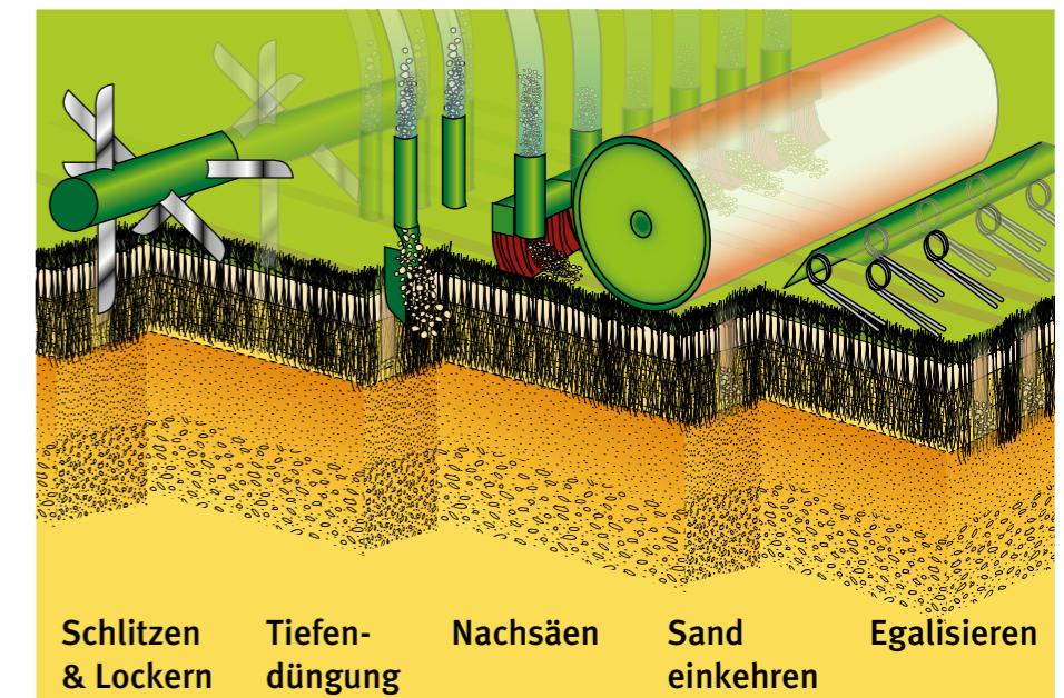
Die 5 Arbeitsschritte mit dem Aeriforce-Gerät.
